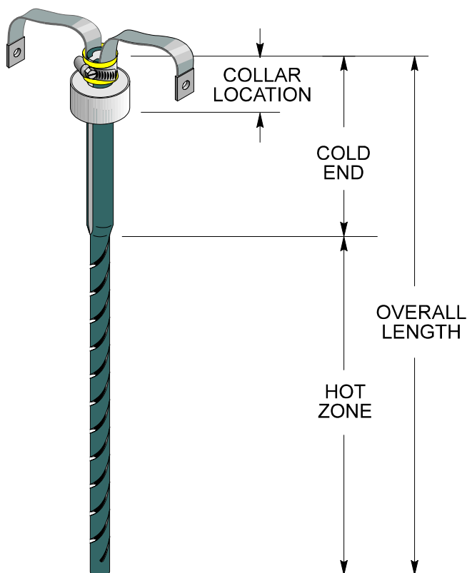
Low-Resistant SEU
